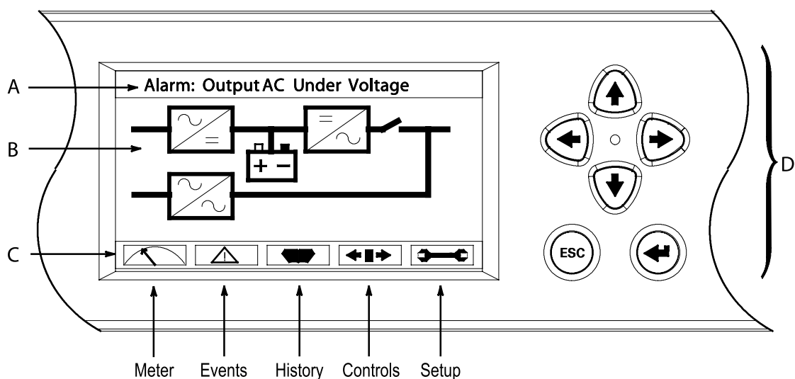
Рис. 6-4: Элементы ЖК-экрана
