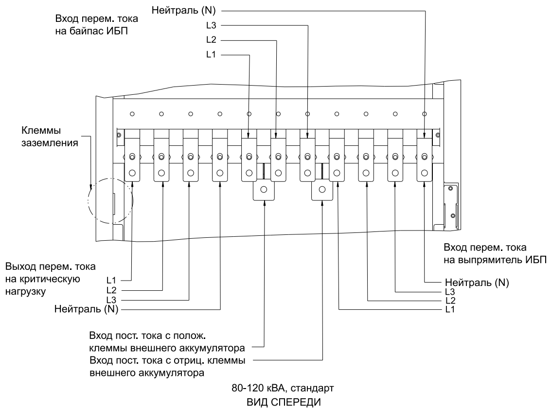
Рис. 4-5: Расположение узлов клемм 80-120 кВА
